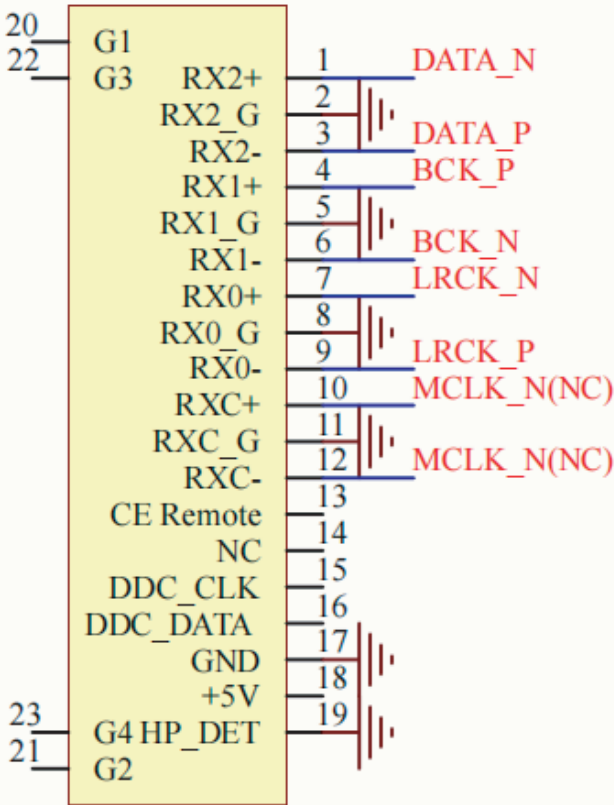
I2S-A I2S(HDMI端子)
